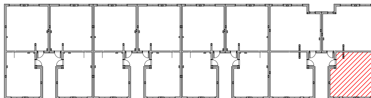
Schemat budynku
